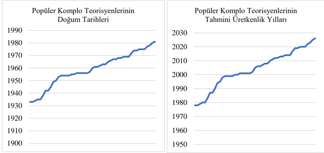
Şekil 1. Teorisyenlerin Doğum Tarihleri ve Üretkenlik Yıllarına İlişkin Projeksiyon
